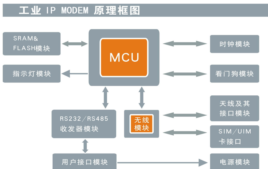
图 1-1 IP MODEM 结构框图
